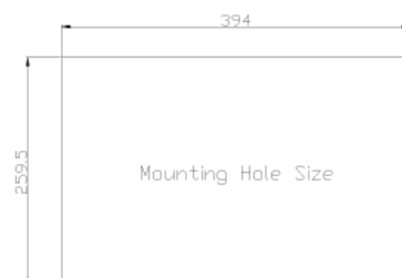
MMI5178B -17''
