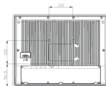
MMI5158B -15''
