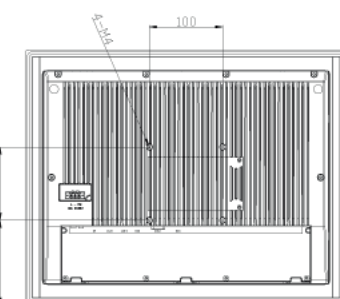
MMI5178B -17''
